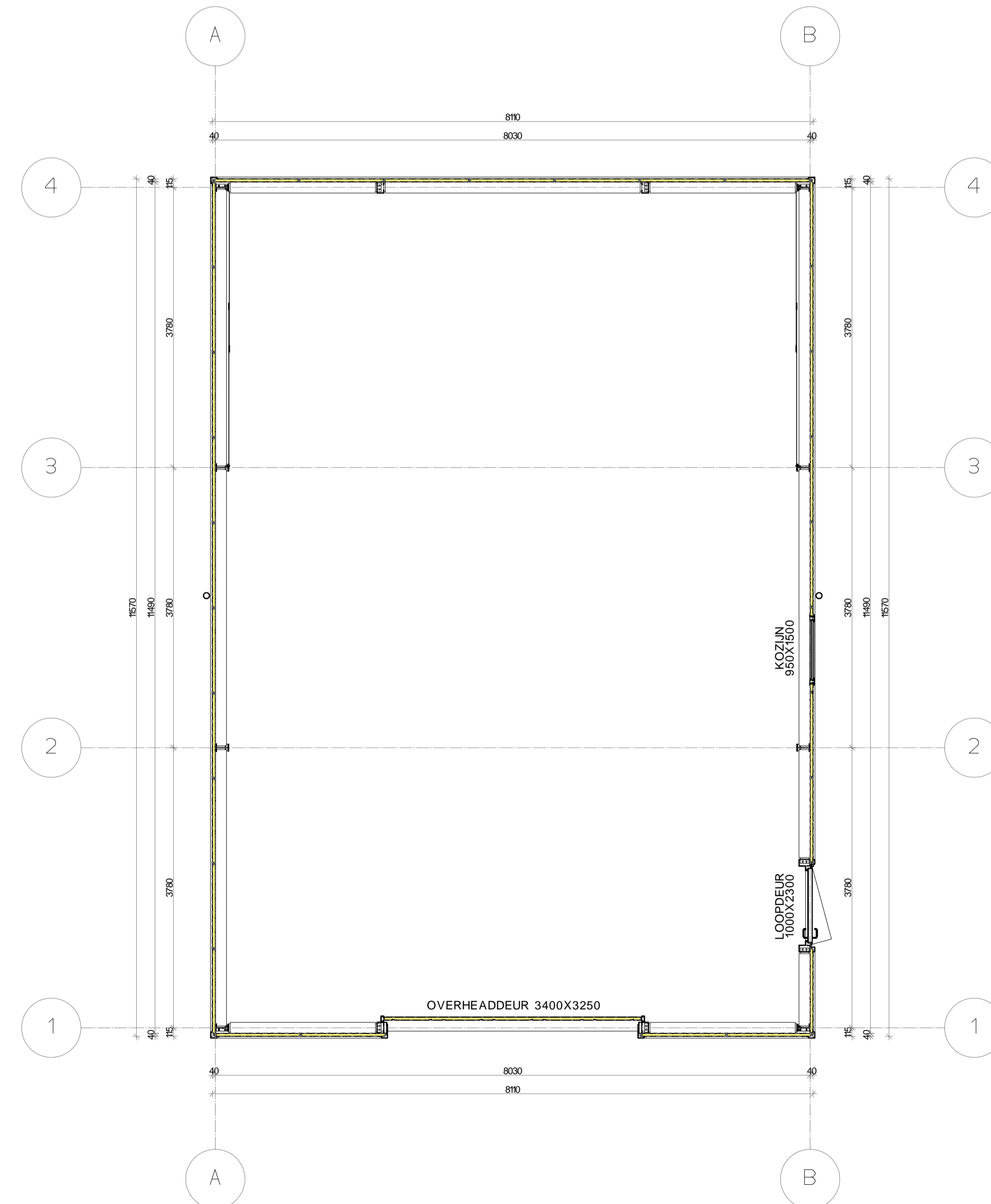
PLATTEGROND
