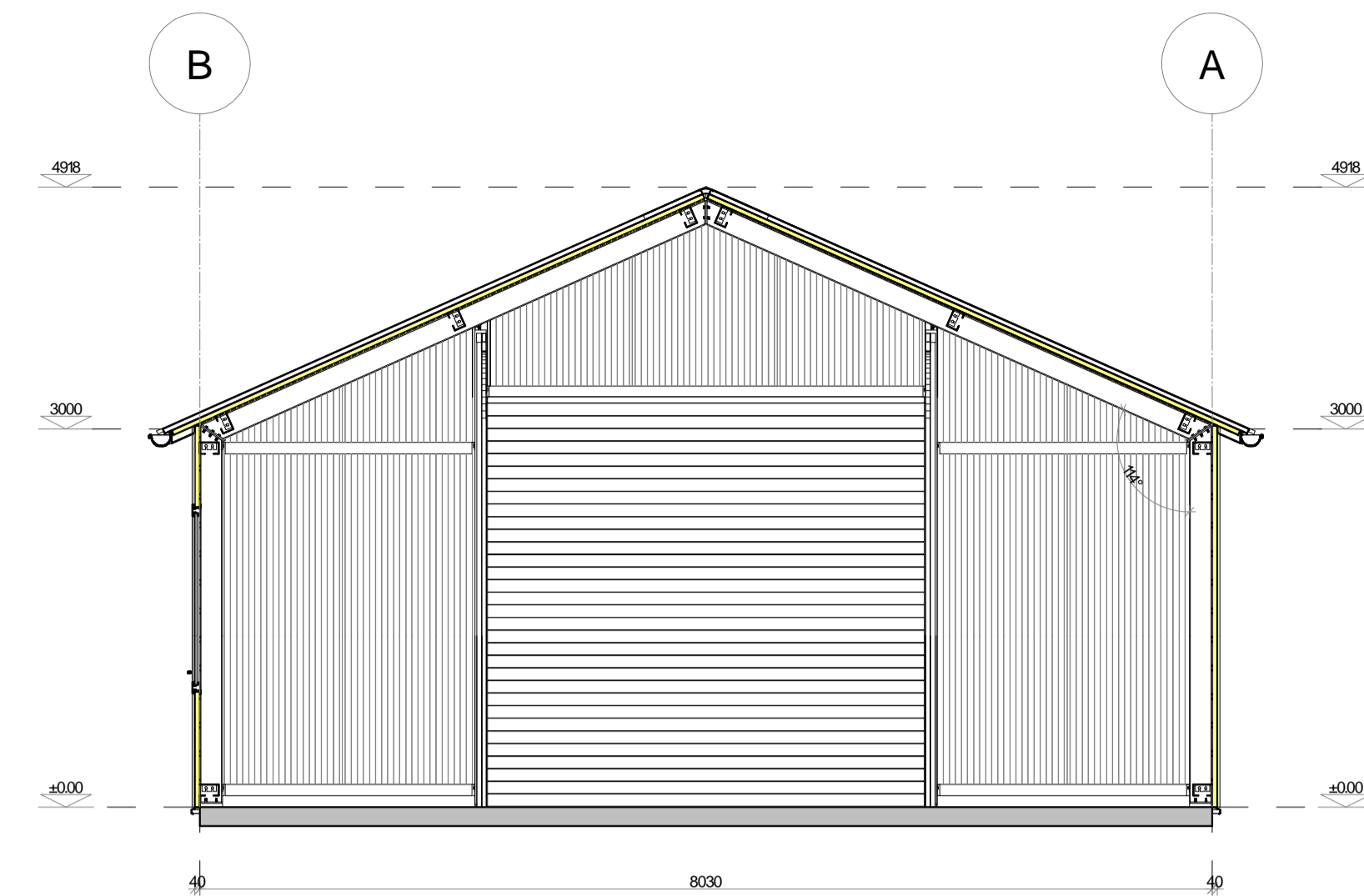
DOORSNEDE
